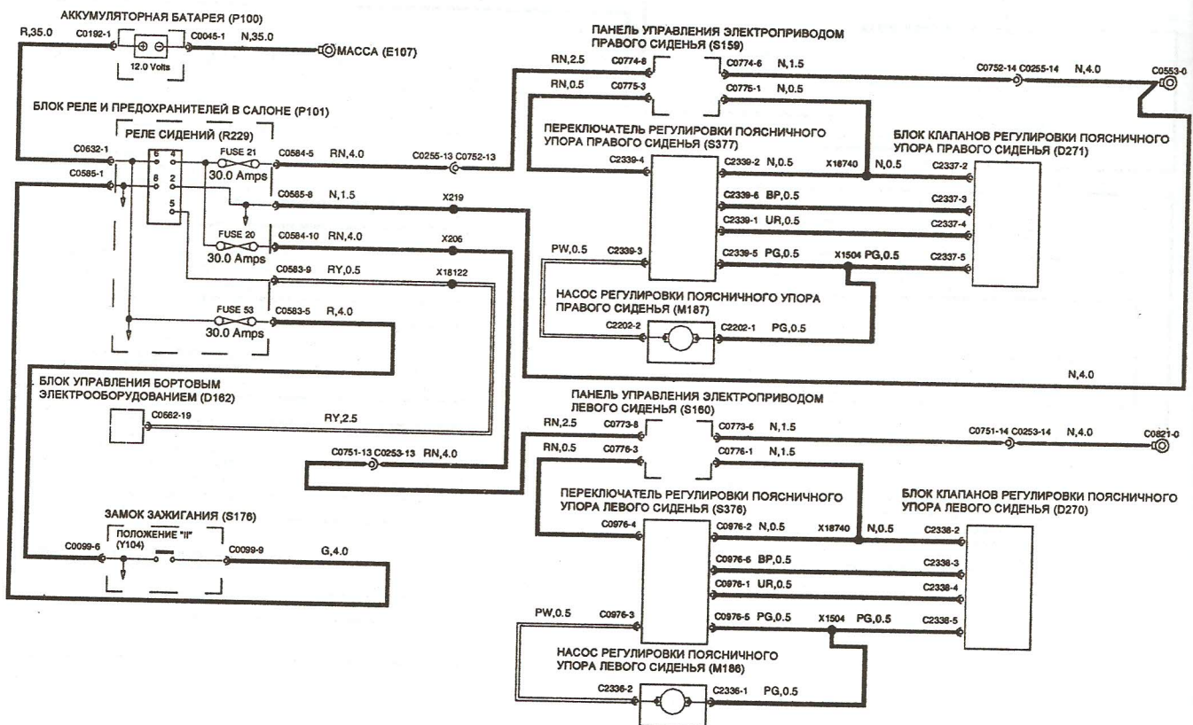
Схема 8-7. ПРИВОД РЕГУЛИРОВКИ ПОЯСНИЧНОГО УПОРА.
