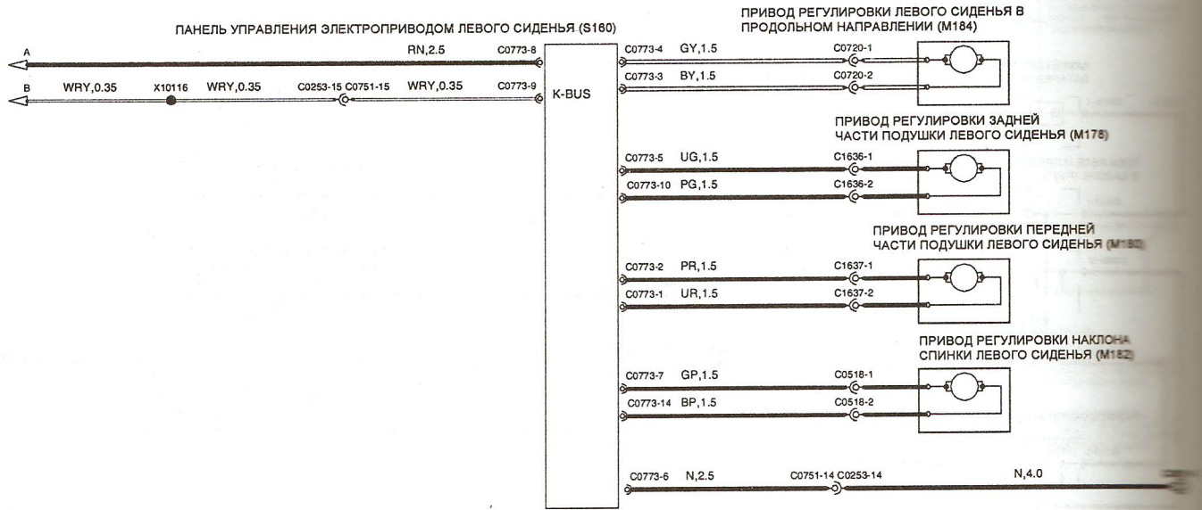
Схема 8-2. ЭЛЕКТРОПРИВОД ПЕРЕДНИХ СИДЕНИЙ.
