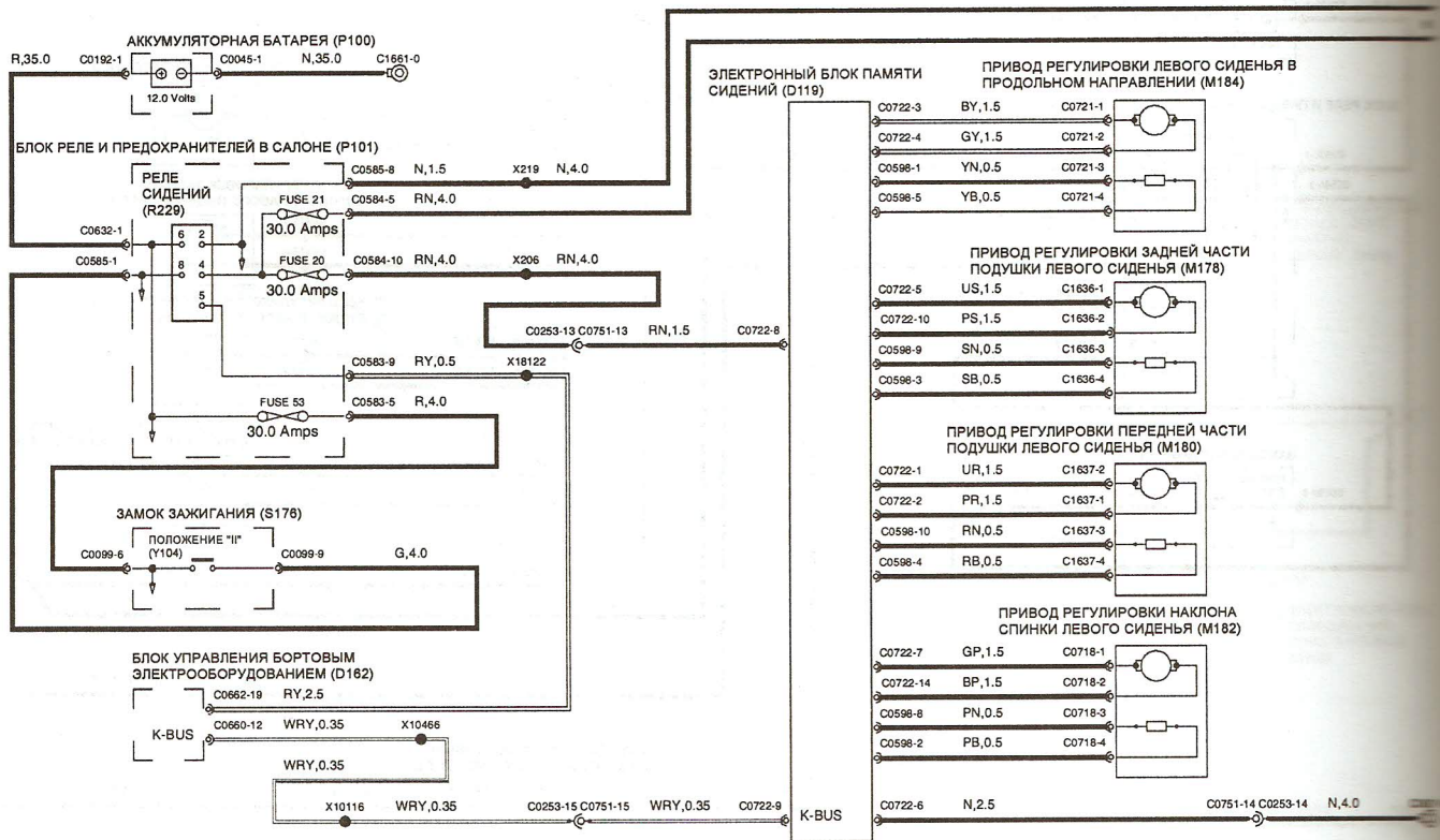
Схема 8-3. СИСТЕМА ПАМЯТИ СИДЕНИЙ.
